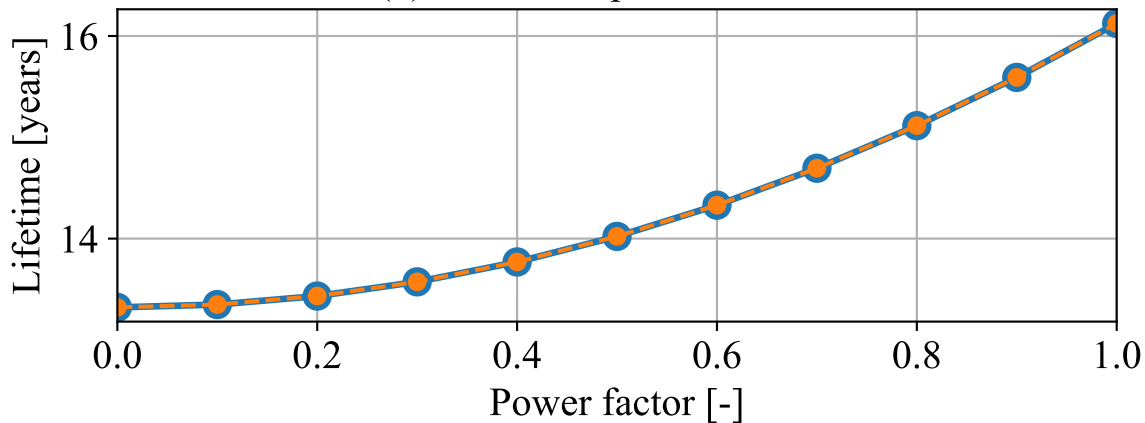
(d) DC-link capacitor lifetime
